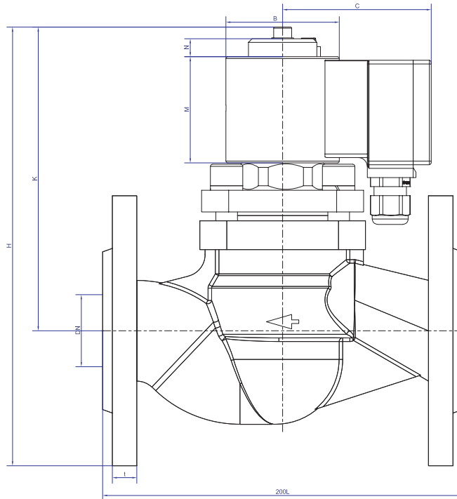
Maßzeichnung Standardausführung Dimensional drawing of standard type
